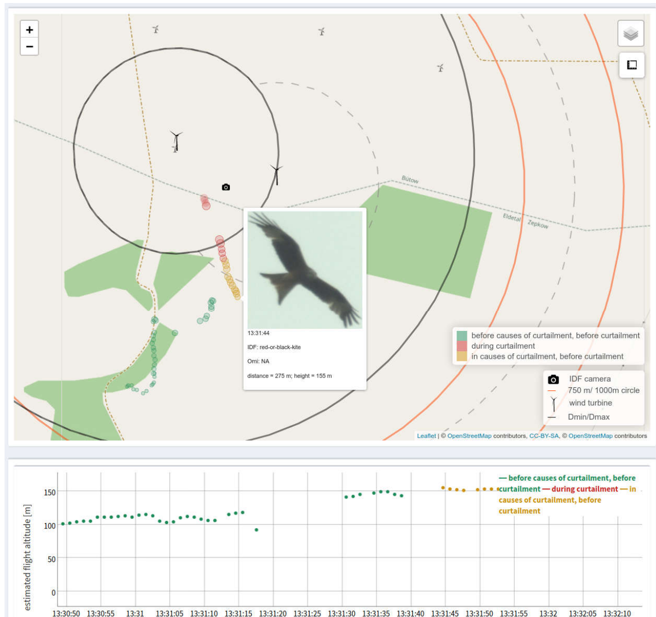
Abbildung 66: Abschaltung beim Eintritt in den inneren Abstandszylinder (innere schwarz Linie) der westlichen WEA am Standort Bütow. Die Abschaltung für diese WEA (rote Punkte) wurde wenige Sekunden nach der Abschaltung für die östliche WEA ausgelöst (siehe Abbildung 65). Standort Bütow, 18.05.2020.
