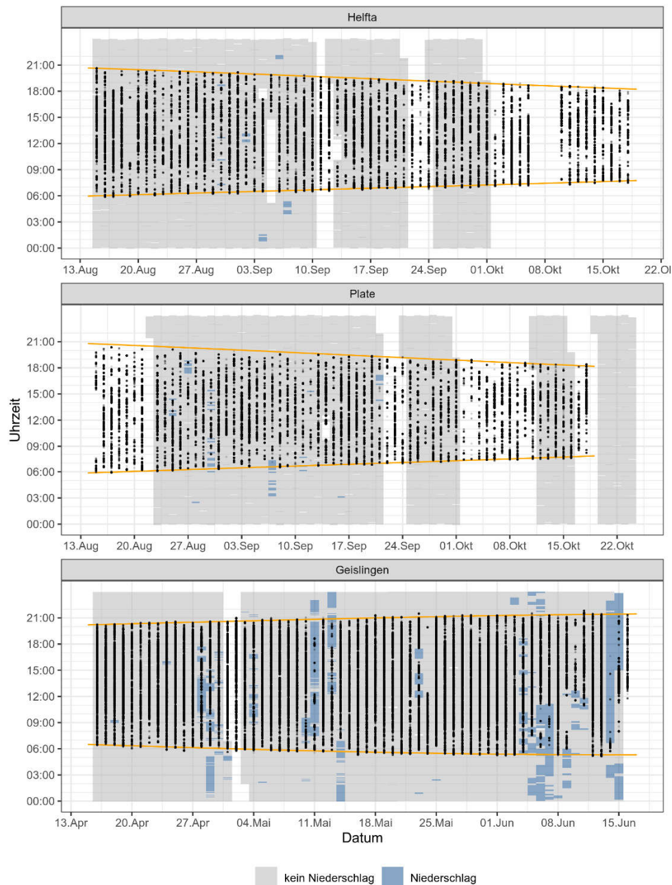
Abbildung 58: Verteilung aller IDF-Erfassungspunkte in Relation zum Niederschlag über den jeweiligen Erfassungszeitraum an den Standorten Helfta (2018), Plate (2018) und Geislingen (2020). Grau gefärbte Zeiträume bedeuten kein Niederschlag, blau gefärbte Zeiträume markieren Niederschlagsereignisse. Für ungefärbte Bereiche innerhalb des Zeitraums der IDF-Erfassungen liegen keine Niederschlagswerte vor. Sonnenaufgang bzw. Sonnenuntergang sind jeweils mit einer orangen Linie gekennzeichnet.
