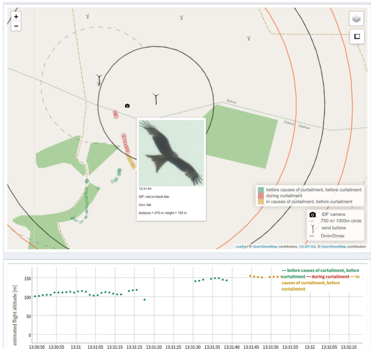
Abbildung 65: Abschaltung beim Eintritt in den inneren Abstandszylinder (innere schwarze Linie) der östlichen WEA am Standort Bütow. Die Abschaltung wurde mit dem ersten Punkt im inneren Abstandszylinder ausgelöst (rote Punkte). Standort Bütow, 18.05.2020.
