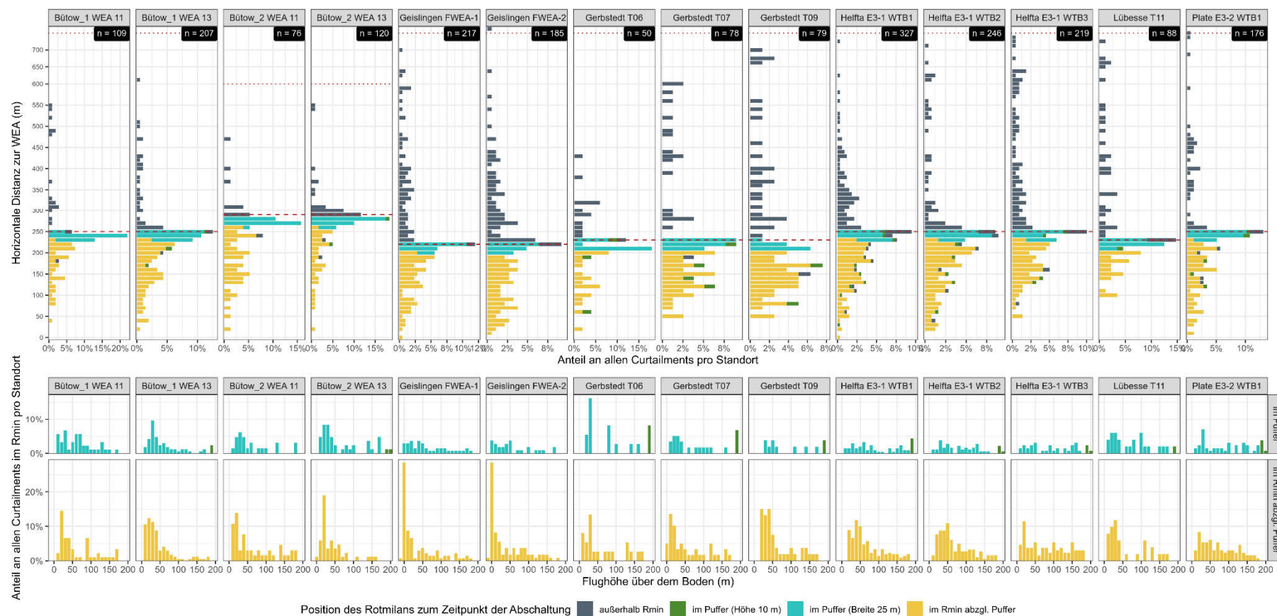
Abbildung 70: Oben: Anteil der Abschalt-Initiierungen in Relation zur Entfernung zu den WEA. Rot gestrichelt sind die jeweils R_{min} und R_{max} . Unten: Anteile der verschiedenen Flughöhen im Moment der Abschalt-Initiierungen an der Gesamtheit aller Abschaltungen im R_{min} , getrennt für das Innere und den Rand des R_{min} (inkl. Puffer)
