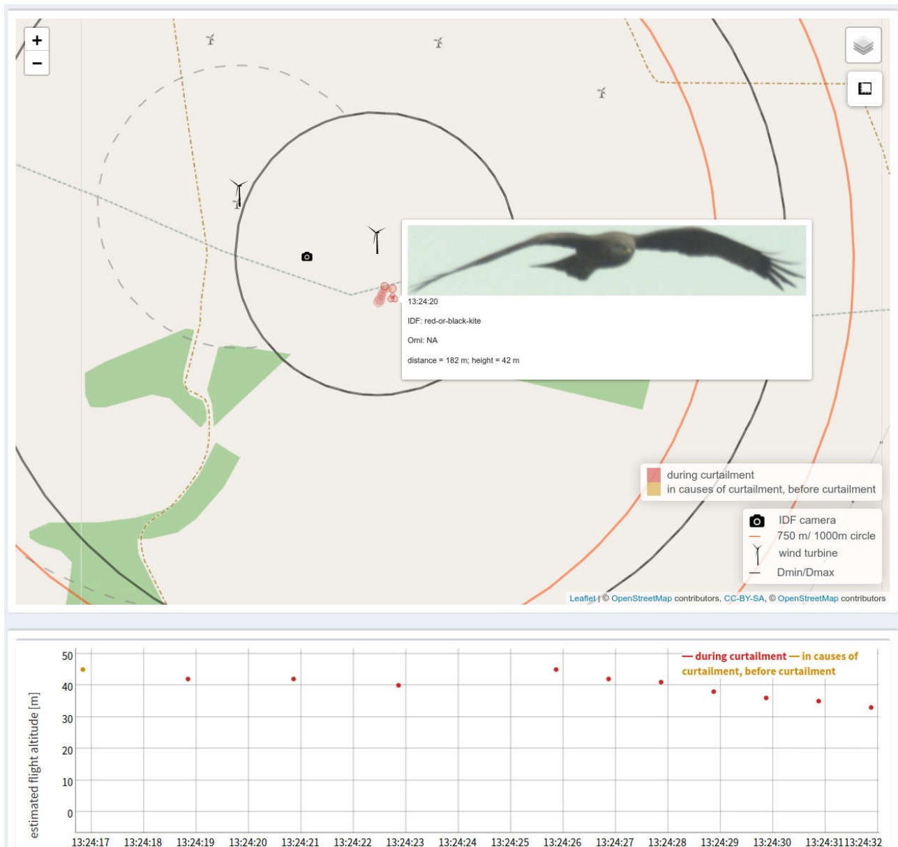
Abbildung 68: Detektion eines Rotmilans im inneren Abstandszyllinders mit unmittelbar folgender Abschaltung am Standort Bütow. Dieser Rotmilan wurde nahe der östlichen WEA in einer Flughöhe von ca. 45 m detektiert (oranger Punkt), beim nächsten Detektionspunkt (rote Punkte) wurde die Abschaltung ausgelöst. Standort Bütow, 18.05.2020.
