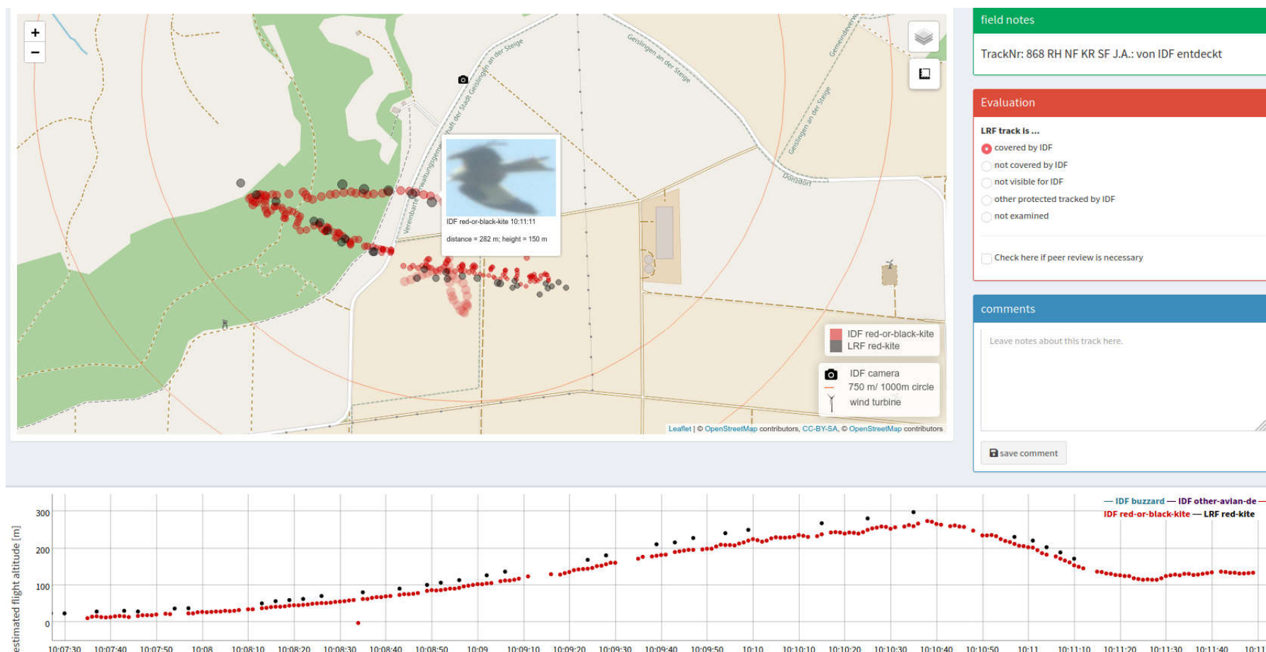
Abbildung 33: Beispiel für die Detektionsbewertung – Kategorie „Erfasst“. Der vom LRF erfasste Rotmilan wurde von IDF ebenfalls erfasst. Standort Geislingen, 06.05.2020.
