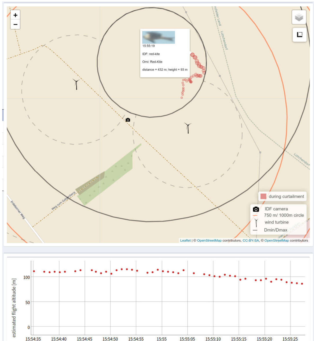
Abbildung 69: Detektion eines Rotmilans im inneren Abstandszyklinders mit unmittelbar folgender Abschaltung am Standort Helfta. In diesem Fall wurde ein Rotmilan in ca. 110 m Flughöhe detektiert, mit dem ersten Punkt der Detektion erfolgt die Abschaltung (nur rote Punkte). Standort Helfta, 10.09.2018.
