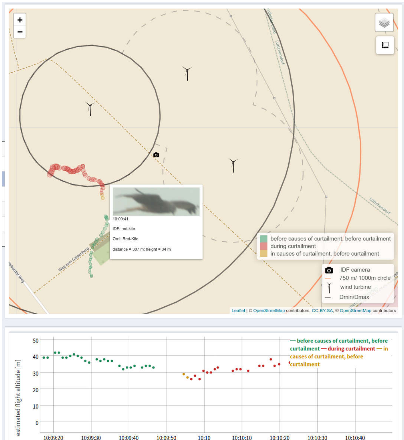
Abbildung 64: Abschaltung im äußeren Abstandszyylinder am Standort Helfta. In diesem Fall löst IDF die Abschaltung kurz vor Erreichen des inneren Abstandszyinders (innere schwarze Linie) aus. Standort Helfta, 24.08.2018.
