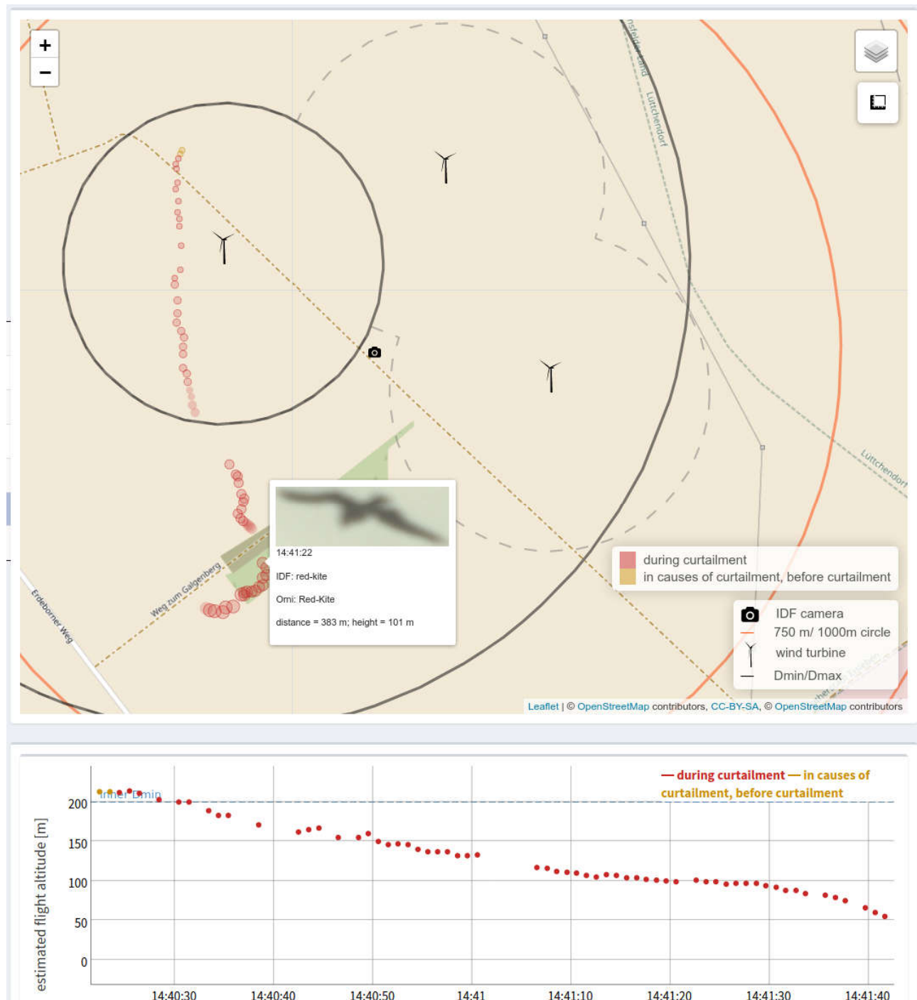
Abbildung 67: Abschaltung oberhalb des inneren Abstandszyllinders am Standort Helfta. In diesem Fall wurde der Vogel oberhalb des inneren Abstandszyllinders (innere schwarze Linie) detektiert und beim Beginn eines Sinkflugs, noch oberhalb der Höhenbegrenzung des inneren Abstandszyllinders (blaue Linie im Höhendigramm), eine Abschaltung ausgelöst. Standort Helfta, 12.09.2018.
