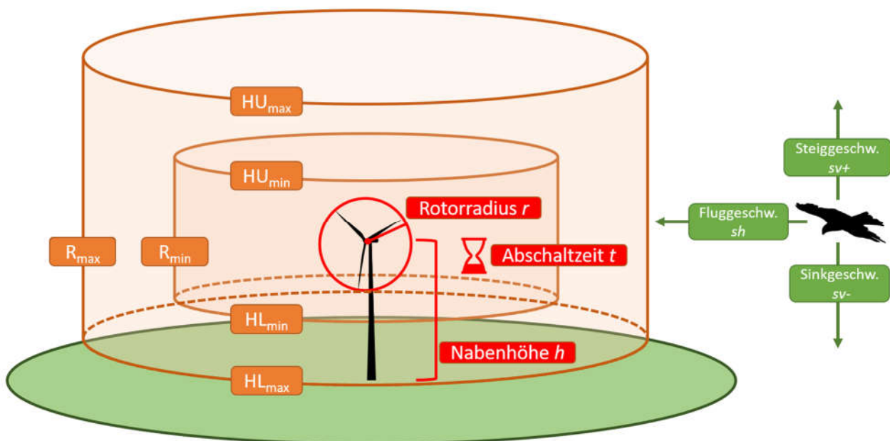
Abbildung 86: Schema zur Dimensionierung der inneren und äußeren Abstandszylinder und den zur Berechnung notwendigen Variablen.
