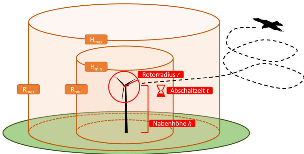
Abbildung 6: Grundlagen des bedarfsgesteuerten Abschaltalgorithmus von IdentiFlight im Rahmen dieser Studie
