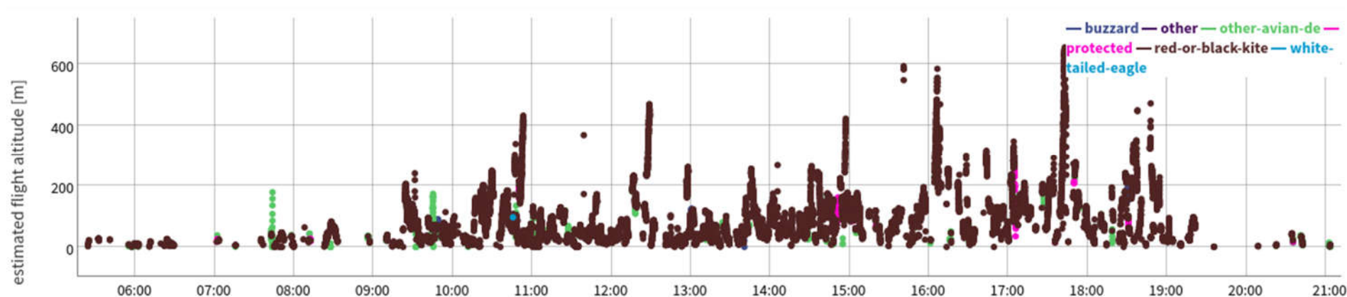
Abbildung 40: Typische Höhenverteilung von Tracks von durch IDF bestimmten Rotmilanen. Gut zu erkennen ist die vertikale Verteilung der Tracks, welche zur Bestimmung der Flughöhen genutzt wurde. Datengrundlage: alle Rotmilanpunkte eines Beispieltages am Standort Geislingen, 01.06.2020.
